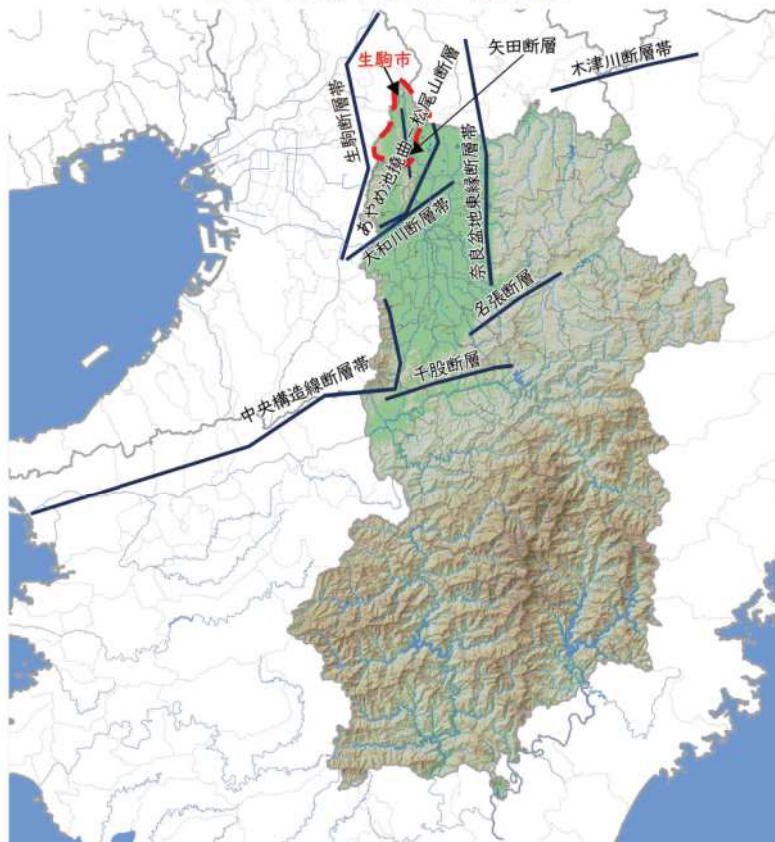
図表 生駒市周辺の断層位置
